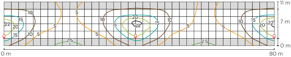
ARREGLO DE 3 LUMINARIAS
